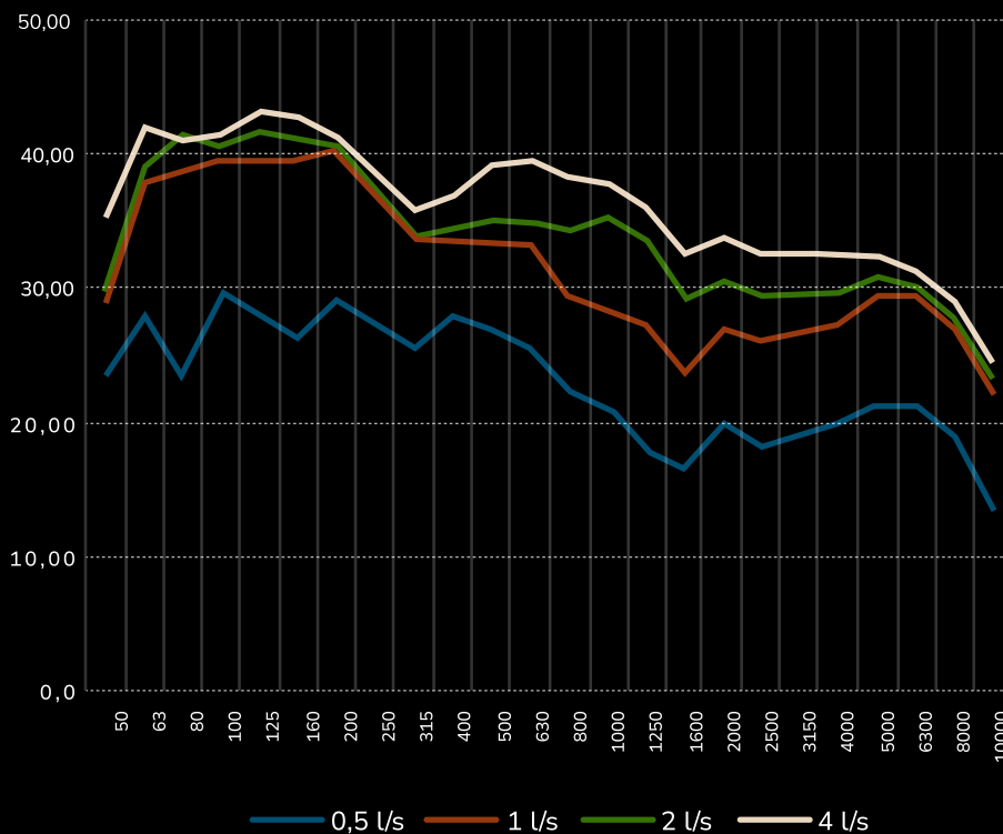
Mitattu ilmaäänitehotaso L_{Wa} [dB]
